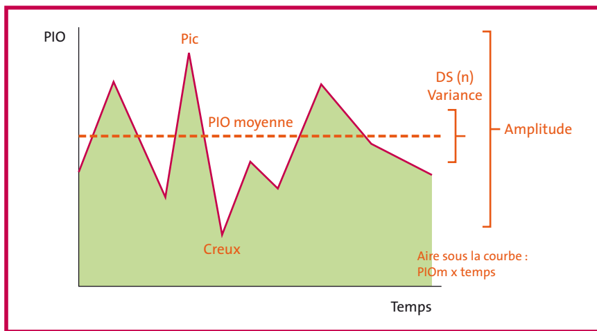
FIG. 1: Fluctuations de la PIO. L'aire sous la courbe de PIO reflète la pression moyenne à laquelle est soumise la tête du nerf optique.
