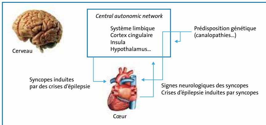
Fig. 1 : Schéma montrant les rapports entre syncopes et crises épileptiques. En particulier une atteinte du central autonomic network (CAN) est à l'origine des réponses neurovégétatives des crises épileptiques qui peuvent comporter des syncopes.
