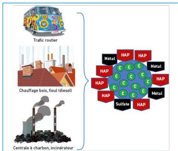
Fig. 1 : Particules fines et ultrafines de combustion: exemple de particule diesel. Le noyau central est composé d'atomes de carbone pur (C), la périphérie de la particule concentre les molécules toxiques. HAP : hydrocarbures aromatiques polycycliques, métaux, sulfates.
