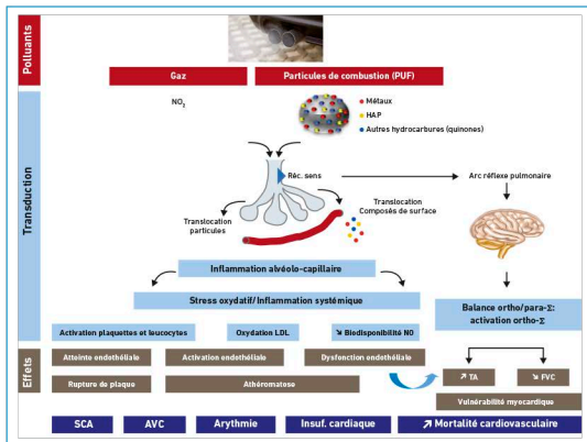
Fig. 3 : Mécanismes physiopathologiques impliqués dans les effets cardiovasculaires de la pollution de l'air. Exemple de la pollution du trafic routier. PUF: particules ultrafines; TA: tension artérielle; FVC: fréquence de variabilité cardiaque; SCA: syndrome coronarien aigu; AVC: accident vasculaire cérébral; HAP: hydrocarbures aromatiques polycycliques; Réc. sens: récepteurs sensitifs; \text{NO}_2 : dioxyde d'azote; \text{O}_2 : ozone; PM: matière particulaire (particules); Insuf. cardiaque: insuffisance cardiaque; \Sigma : système sympathique; ortho- \Sigma : système orthosympathique; para- \Sigma : système parasymphathique.
