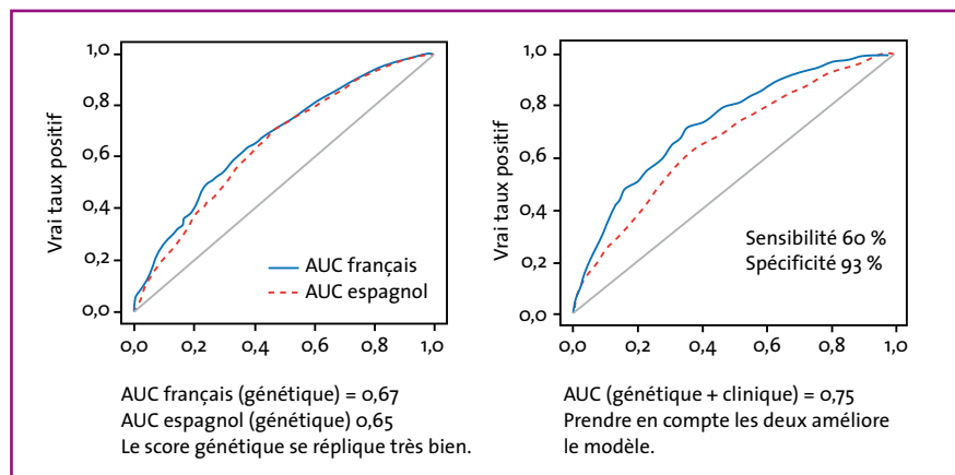
FIG. 2 : Prédiction du risque de mélanome par le test Melapred. À gauche, prédiction du risque de mélanome par les marqueurs génétiques. Cette prédiction, mesurée par l'aire sous la courbe (AUC) se réplique bien entre les populations. À droite, la prédiction mesurée par le test Melapred est beaucoup plus performante (courbe noire, AUC = 0,75).
